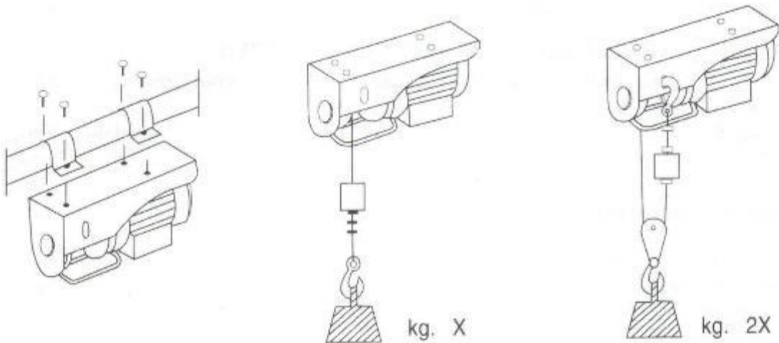
Рисунок 2. Установка тали.
